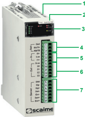
PMESWT0100
